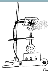
かりょくはつでんじょうもけい 火力発電所模型
