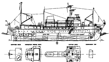
図3 調査船のレイアウト
