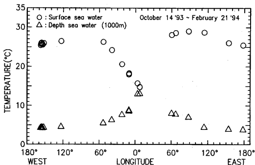
図30 経度と表層と深層の温度差
