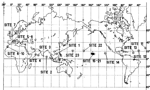
図1 世界のエネルギー源調査海域
