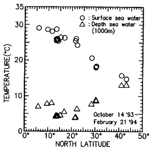
図29 緯度と表層と深層の温度差の関係
