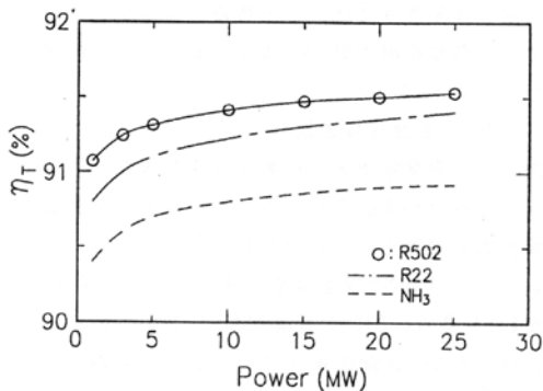
図4 タービン効率
