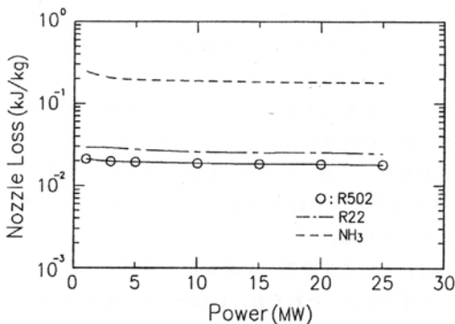
図6 ノズル損失
