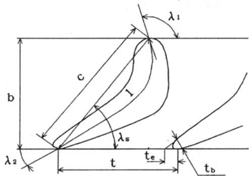
図2 翼の形状
