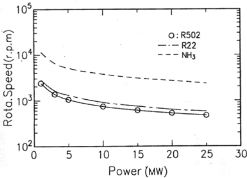
図 12 回転数
