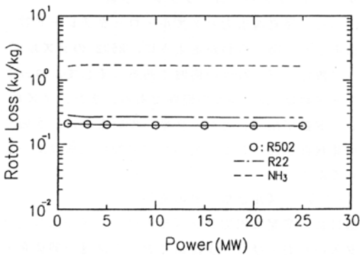
図7 ロータ損失
