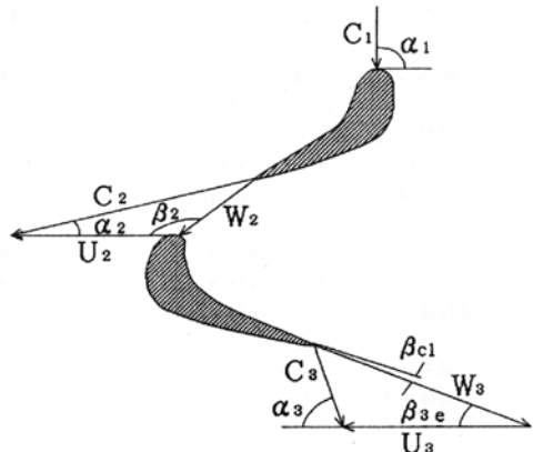
図3 速度三角形
