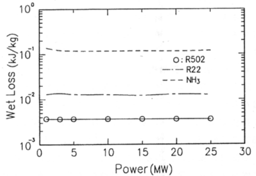
図 10 湿り損失
